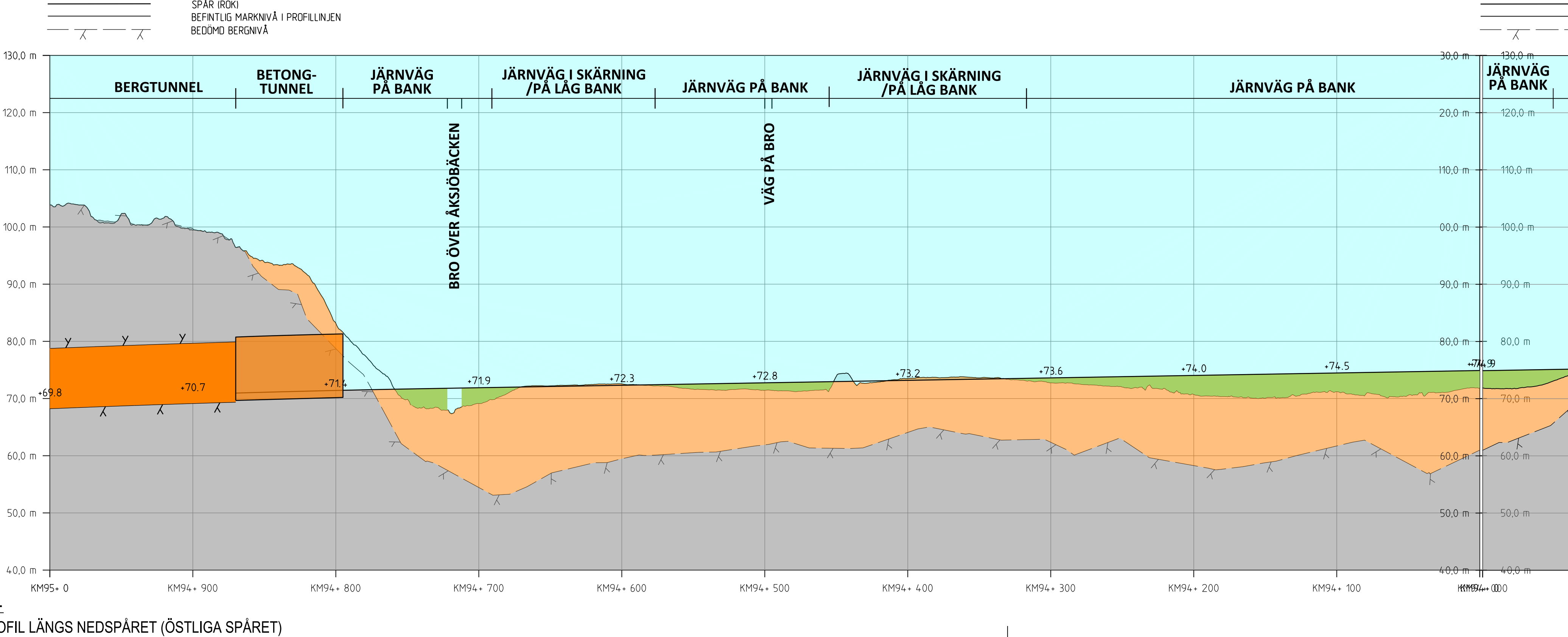
PROFIL LÄNGS NEDSPÅRET (ÖSTLIGA SPÅRET)
